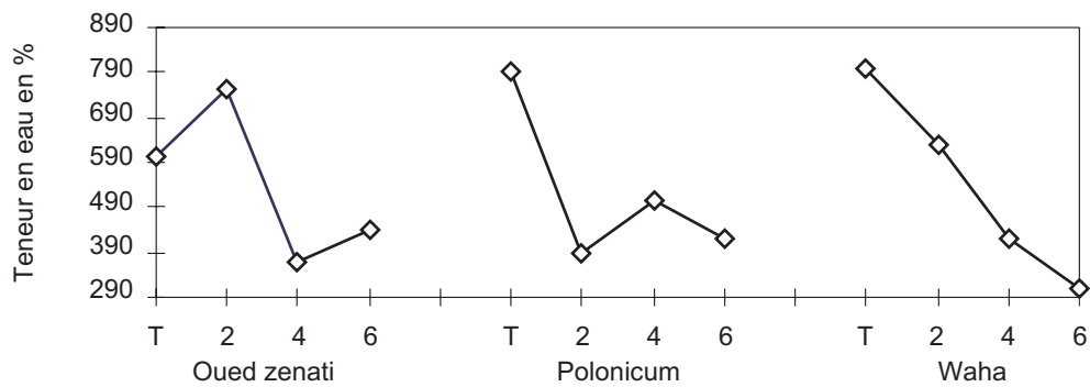
Fig. 1. La teneur en eau des trois variétés de blé dur au stade 4-5 feuilles selon les concentrations en NaCl.
