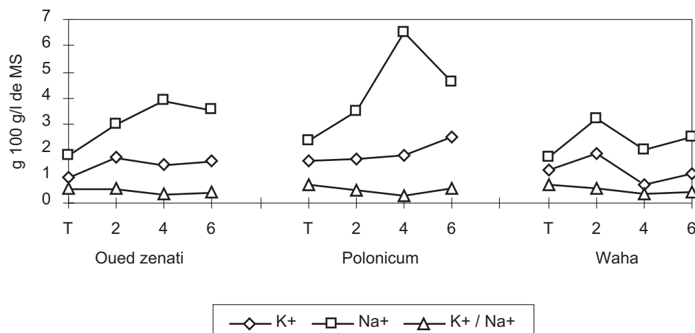
Fig. 2. La teneur d'ions minéraux foliaires de trois variétés de blé dur selon les concentrations en NaCl.
