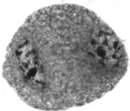
Fig. 8. Prophase II.
