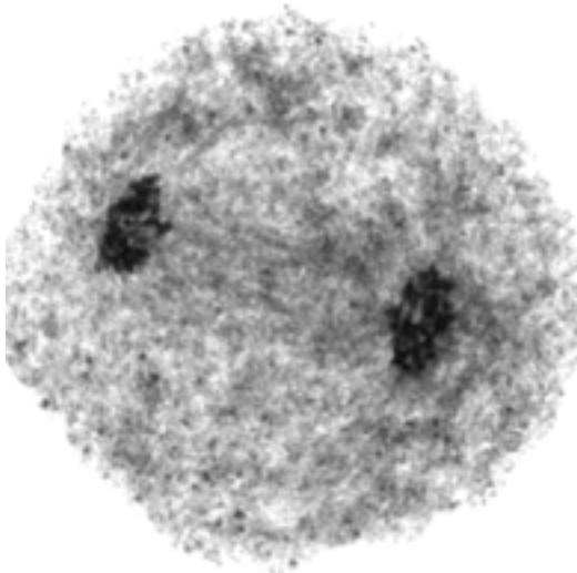
Fig. 7. Telophase I.
