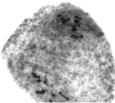
Fig. 9. Metaphase II.
