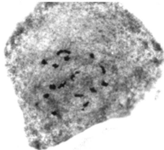
Fig. 4. Metaphase I.
