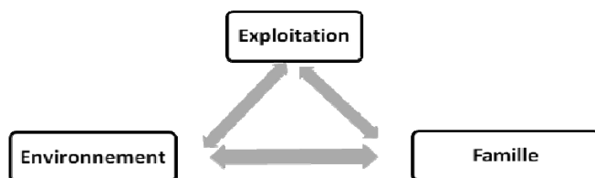
Figure 2. Système exploitation-famille-environnement
