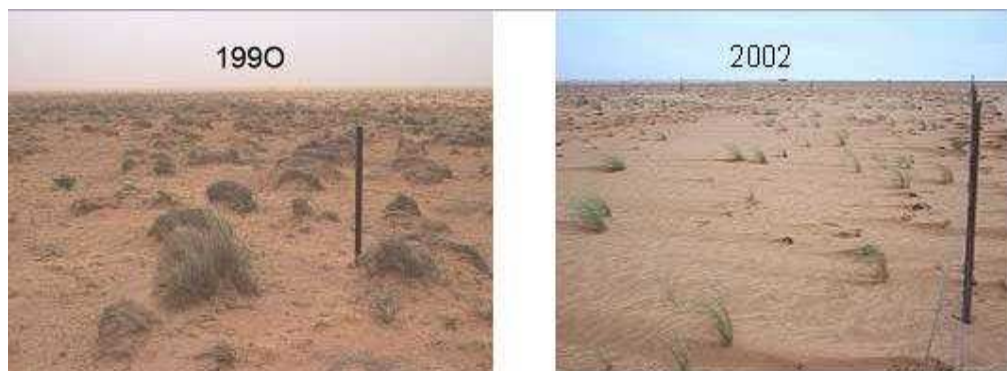
Figure 3.3. Dégradation des steppes à alfa de 1990 à 2002
